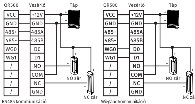
RS485 kommunikáció
